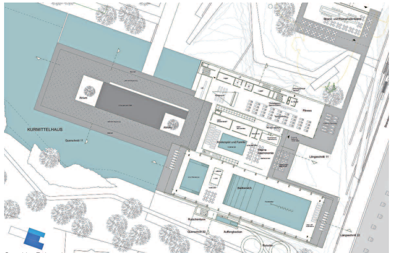
Grundriss Erdgeschoss
