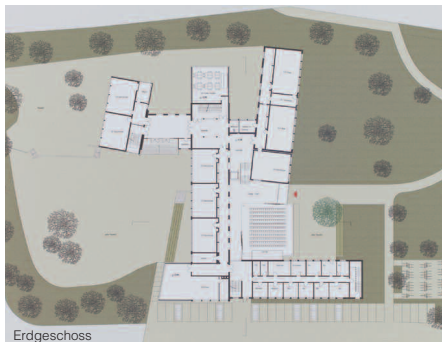
Erdgeschoss
