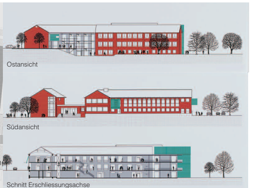
Schnitt Erschliessungsachse
