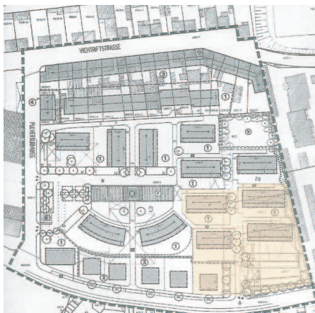
Bebauungsplan
