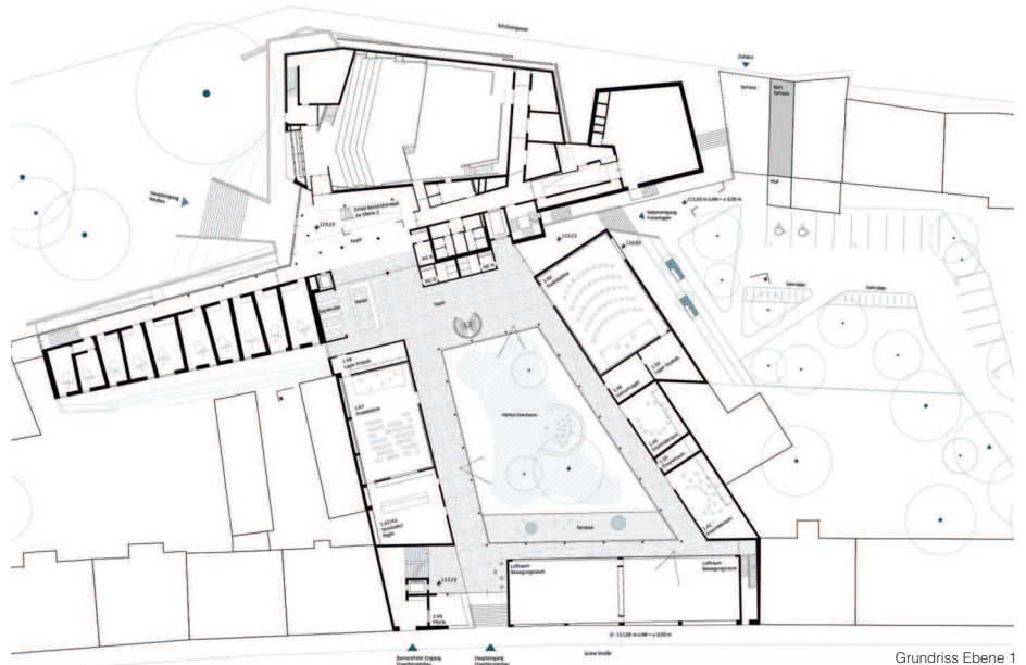
Grundriss Ebene 1
