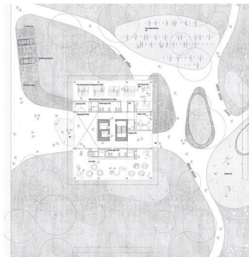
Grundriss Erdgeschoss
