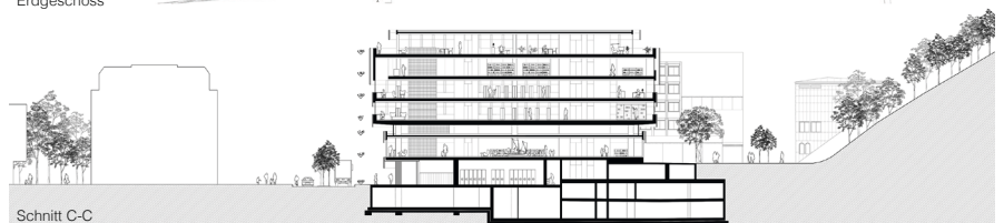
Schnitt C-C
