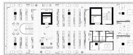
1. Obergeschoss
