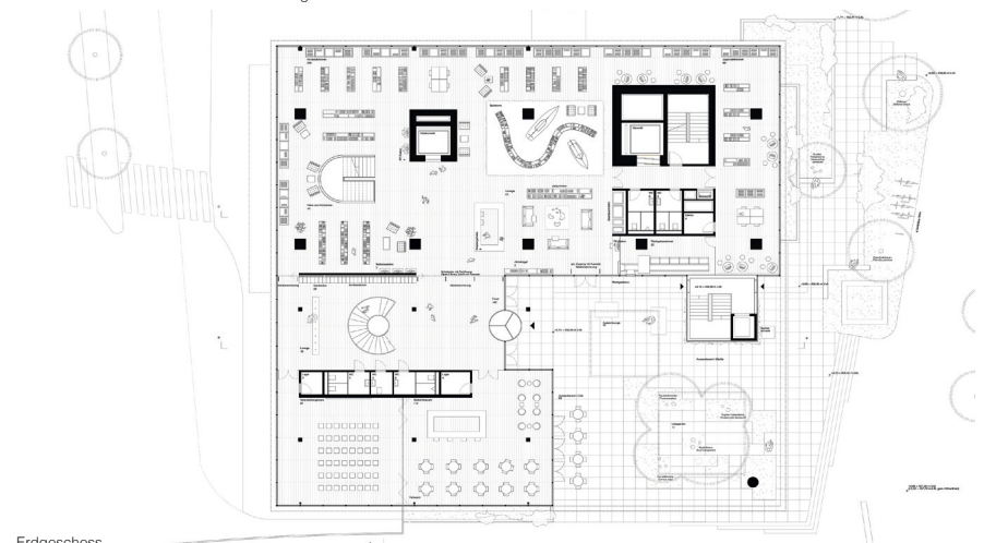
Erdgeschoss
