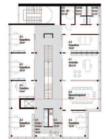
Grundriss 1.OG
