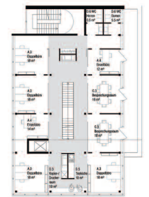
Grundriss 3.OG
