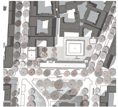
Lageplan
