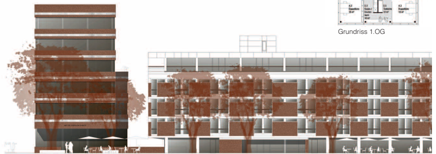
Ansicht Süd
