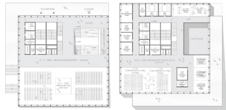
1. Obergeschoss
