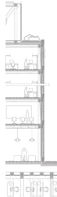
Fassadendetail
