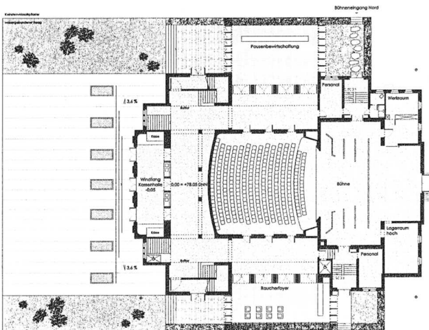
Erdgeschoss 1. Preis
