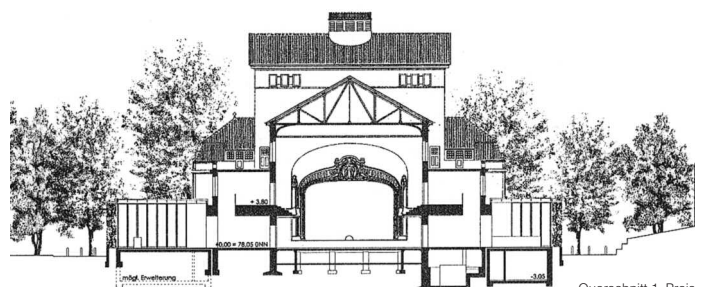
Querschnitt 1. Preis
