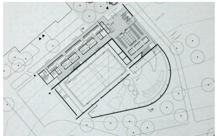
1. Preis: Grundriss Eingangsebene
