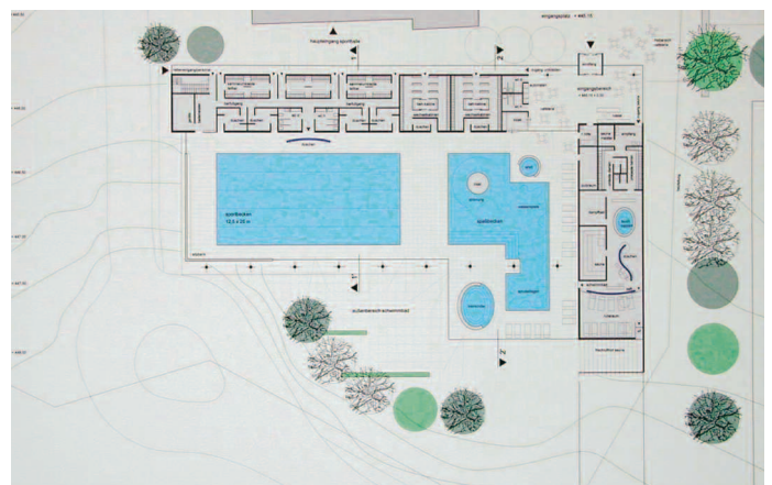
3. Preis: Grundriss Eingangsebene
